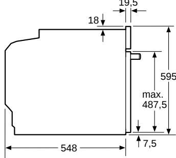
PROIEZIONE LATERALE
