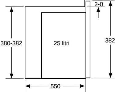
PROIEZIONE LATERALE
