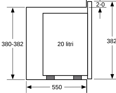
PROIEZIONE LATERALE
