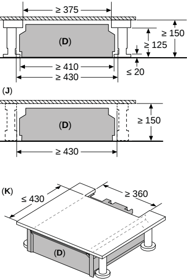
Vista frontale
