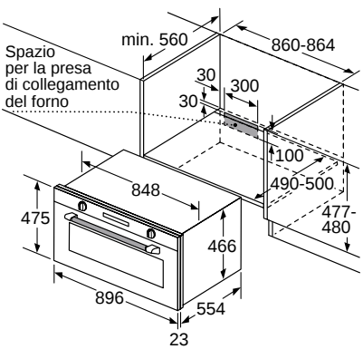
INCASSO SOTTOPIANO
